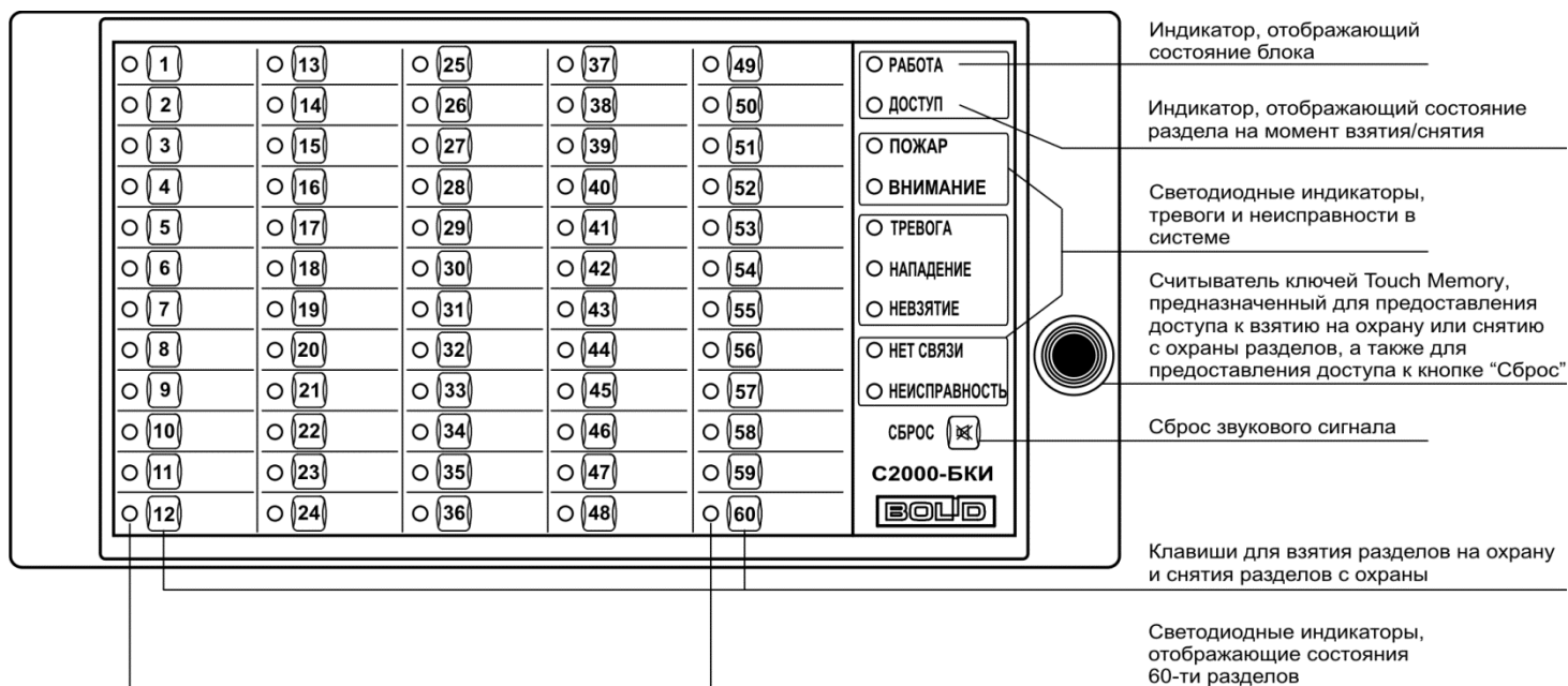
Рисунок 3.10. Внешний вид, органы индикации и управления блока «С2000-БКИ»
