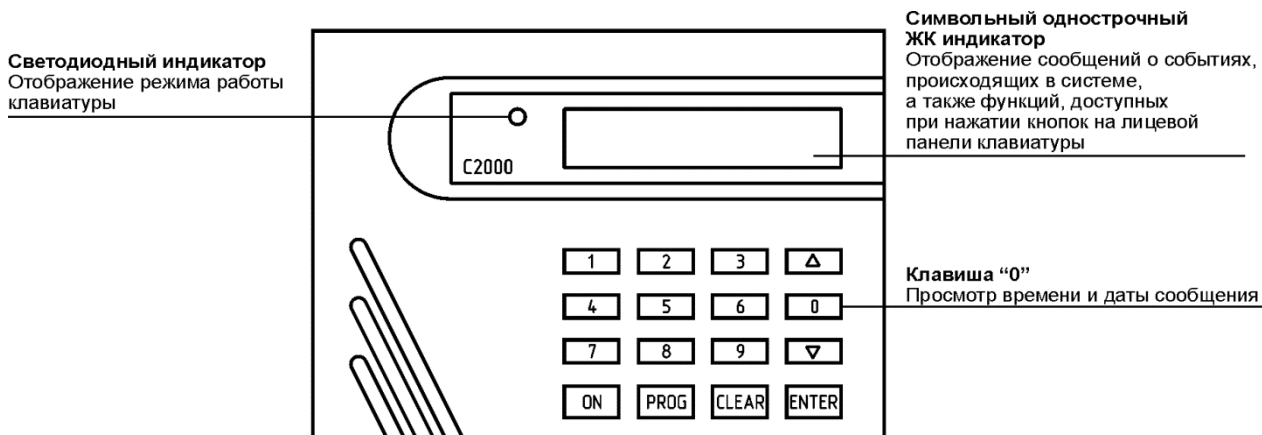
Рисунок 3.2. Внешний вид, органы индикации и управления пульта С2000
