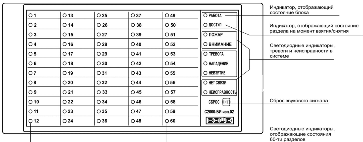
Рисунок 3.9. Внешний вид, органы индикации и управления блока С2000-БИ исп.02
