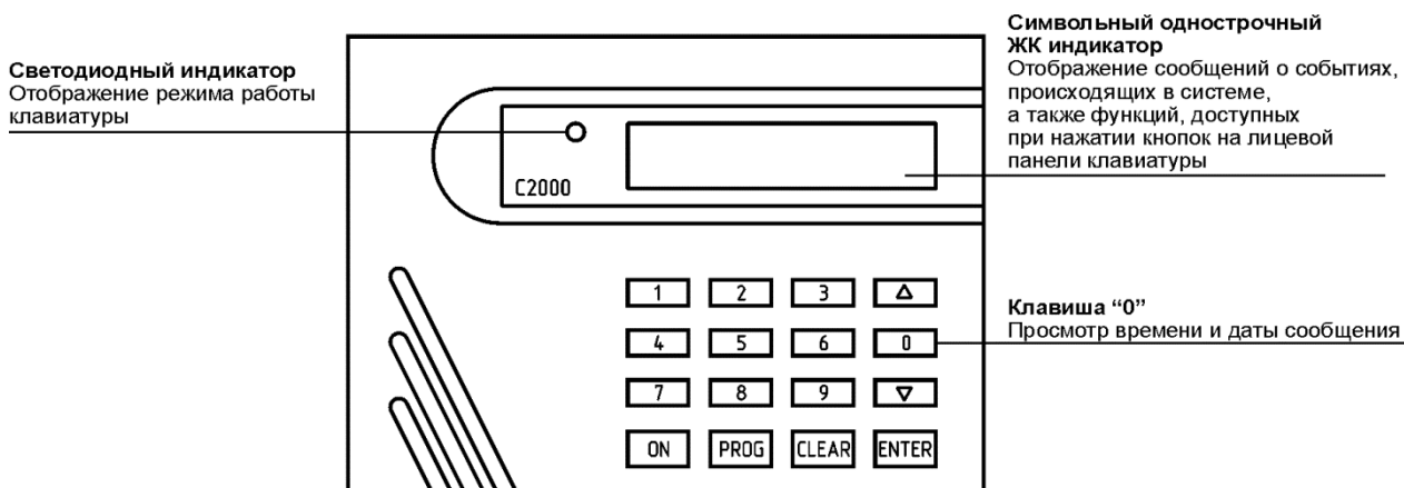
Рисунок 3.6. Внешний вид, органы индикации и управления клавиатуры С2000-К
