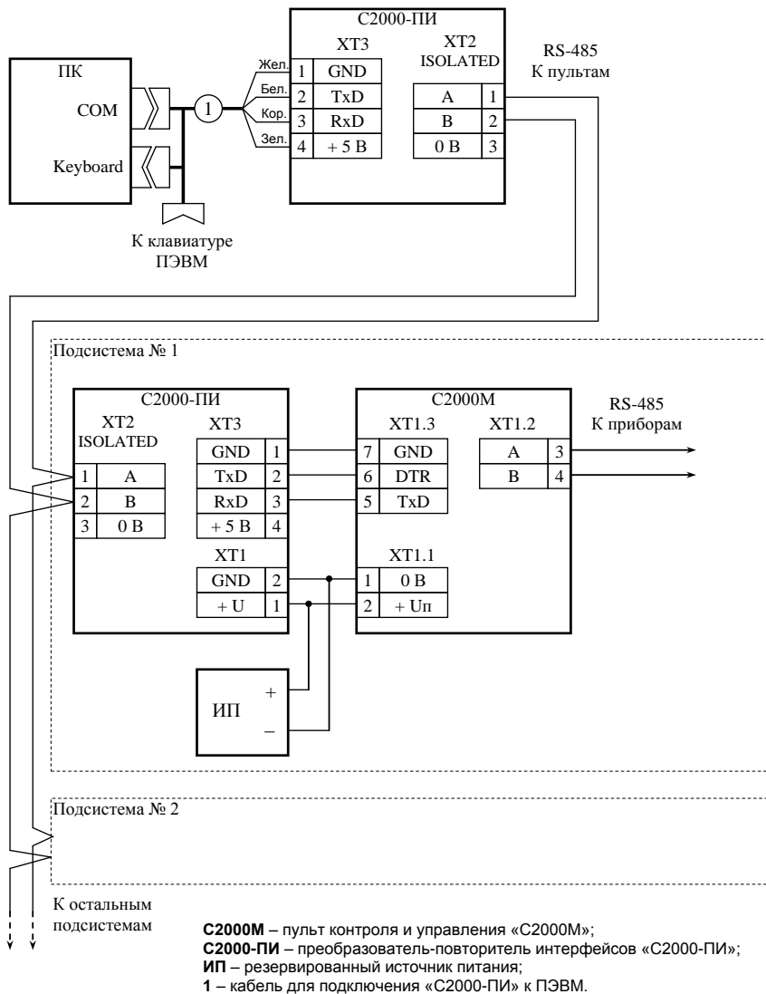
Рис.4. Схема подключения нескольких пультов С2000М (С2000) к персональному компьютеру гальванической изоляцией интерфейса RS-485
